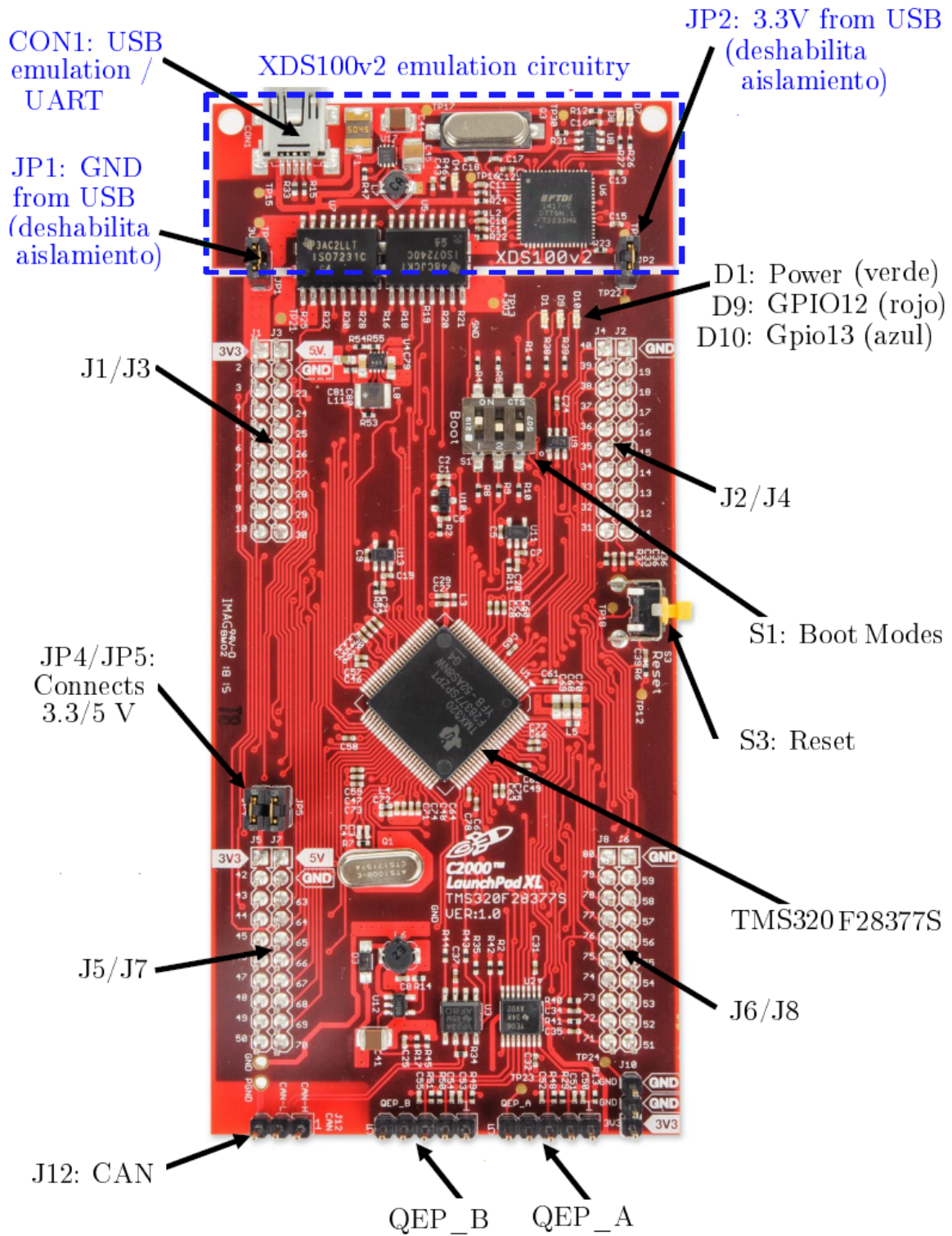
Figura 3.1: Tarjeta LaunchPad Delfino.
