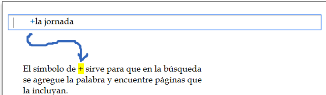
Figura 8. Comando +
