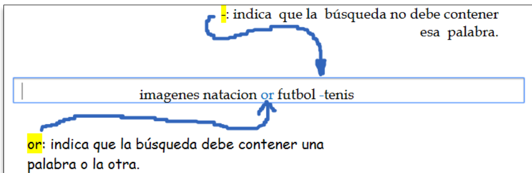
Figura 6. Comando or
