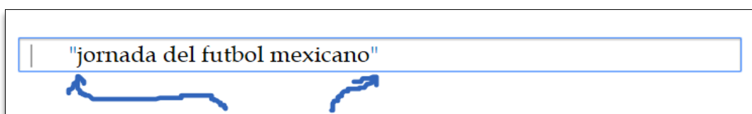
Figura 7. Comando comillas
