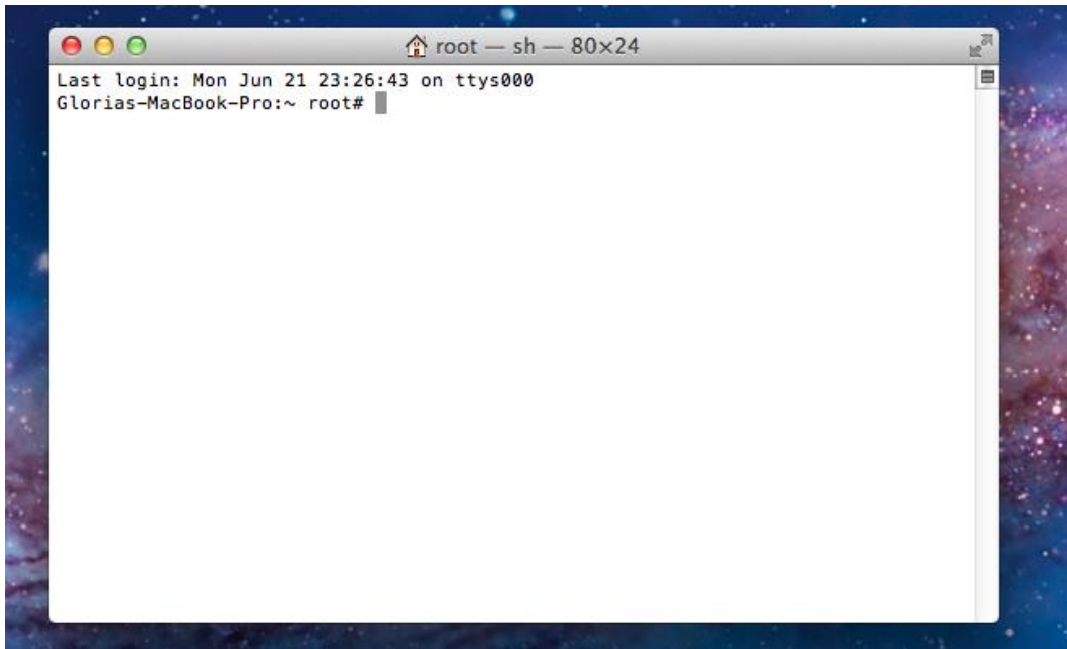
Figura 4: Terminal
