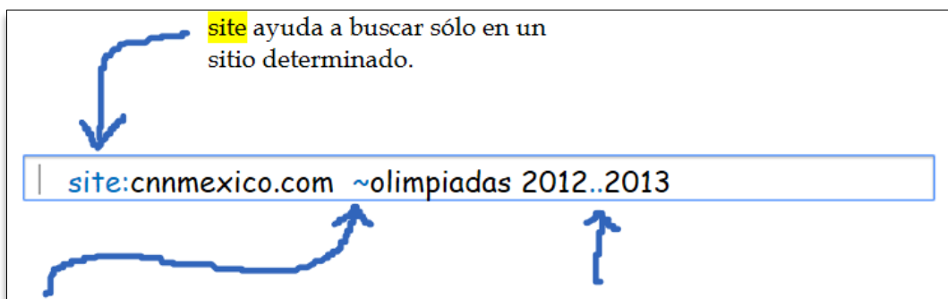
Figura 9. Comando Define
