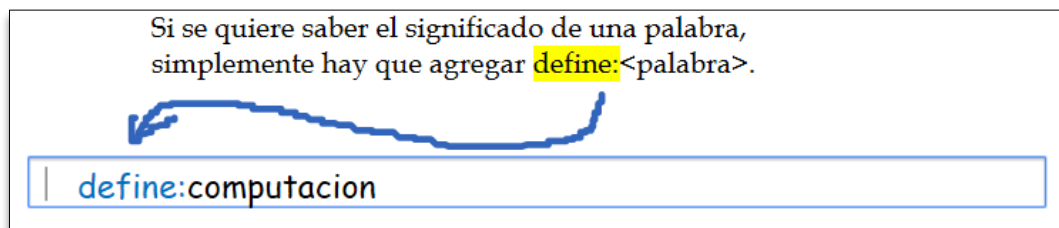
Figura 8. Comando +
