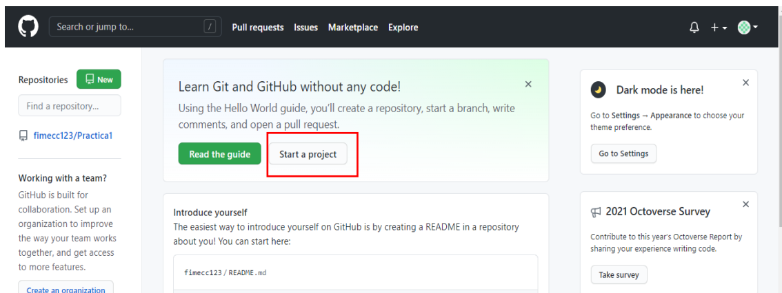
Figura 22. Iniciar proyecto
