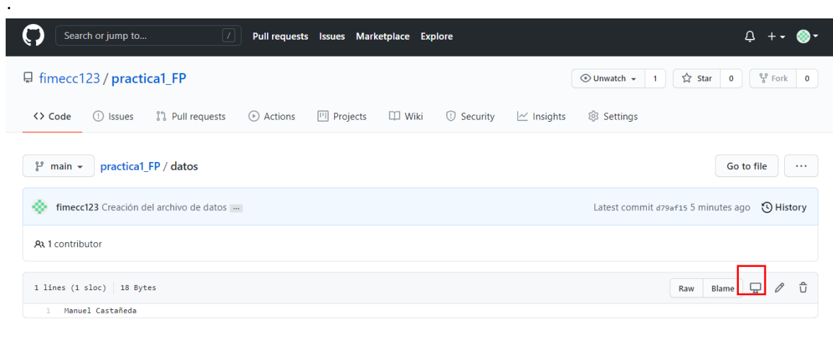
Figura 29. Editar archivo
