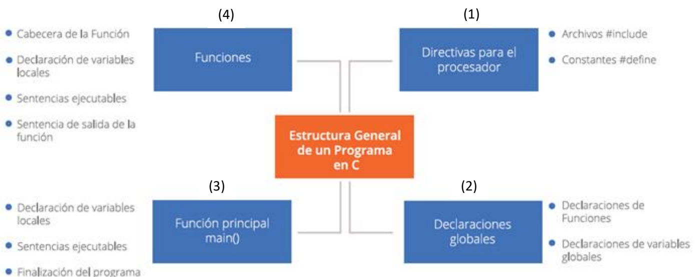
Figura 4: Estructura General de un programa en C
